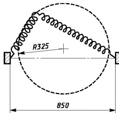
Рисунок 2 — Схема установки для испытания износоустойчивости спиральных шнуров
