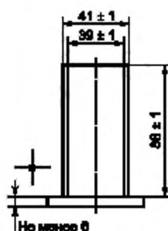
Рисунок 1 — Мерный стакан емкостью 100 \text{ см}^3
