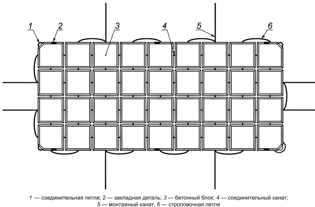
Рисунок 1 — Гибкая бетонная плита, тип 1 (ГБП-1)
