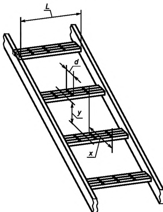
d — ширина горизонтальной плоскости ступеней или перекладин; L — длина ступеней или перекладин кровельной лестницы; x — расстояние между двумя смежными ступенями или перекладинами кровельной лестницы в горизонтальной проекции; y — расстояние между двумя смежными ступенями или перекладинами кровельной лестницы (высота ступенек или перекладин) в вертикальной проекции
