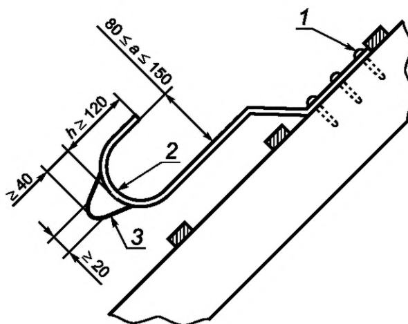
1 — крепеж; 2 — основание крюка; 3 — закрытая петля
