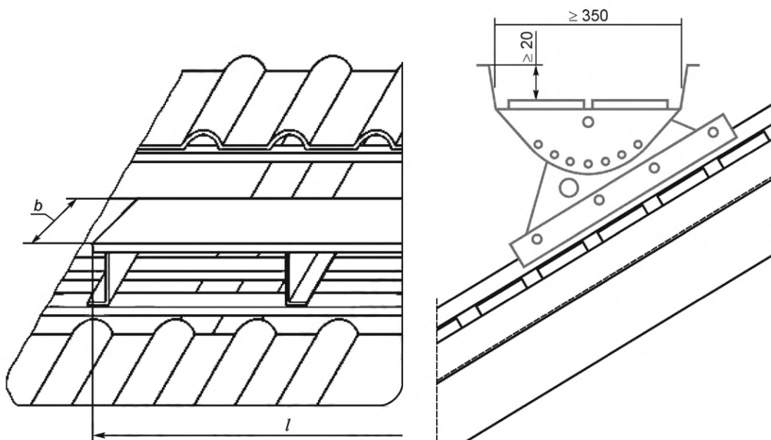
Рисунок 3 — Кровельный мостик
