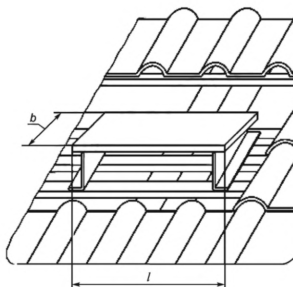
Рисунок 4 — Кровельная ступень
