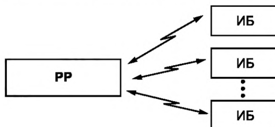
Схема радиального подключения устройств систем беспроводных объектов охранной сигнализации
