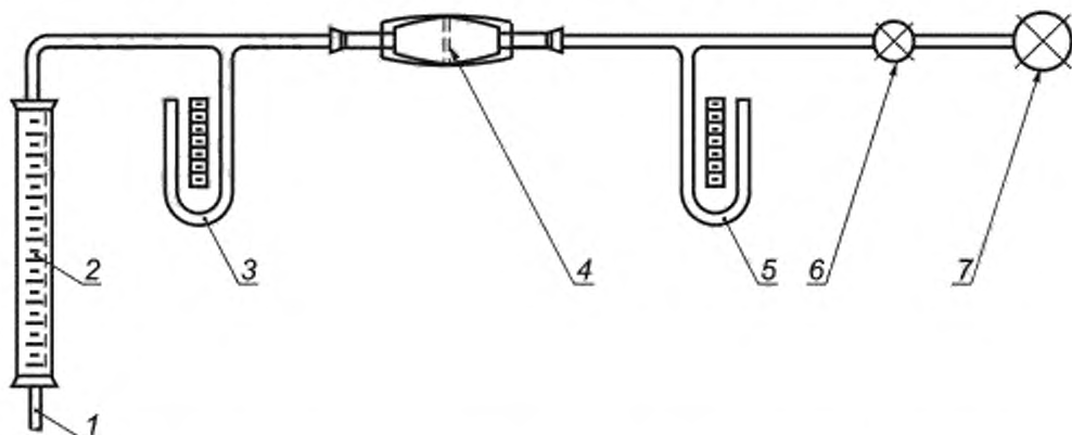
1 — воздушозаборник; 2 — расходомер; 3 — манометр М1; 4 — фильтрующий материал; 5 — манометр М2; 6 — клапан; 7 — вакуумный насос
