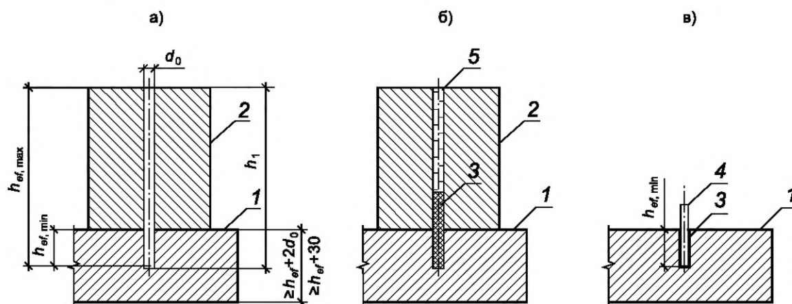
а) бурение отверстия на требуемую глубину h_1 ; б) очистка и заполнение клеевым составом; в) удаление дополнительного блока и установка стального элемента анкера; 1 — основание; 2 — дополнительный бетонный блок; 3 — клеевой состав; 4 — установленный стальной элемент анкера; 5 — заполнение водой (при необходимости)
