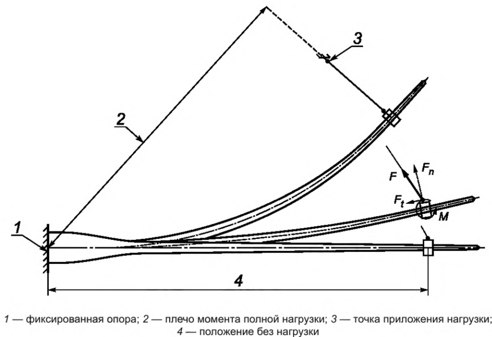
Рисунок F.1 — Влияние приложенных нагрузок на деформацию и угловое искривление лопасти
