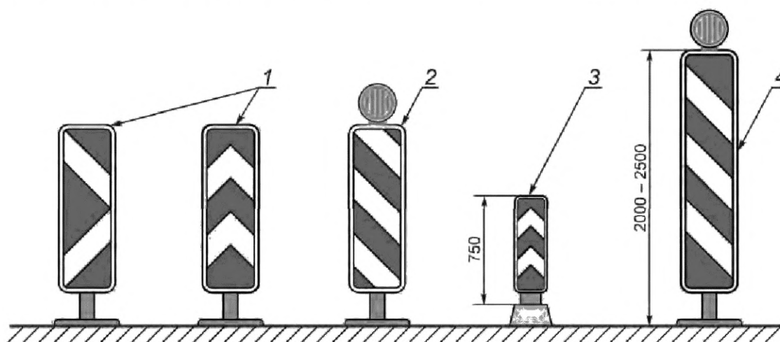
1 — дорожная пластина со стрелами; 2 — дорожная пластина в сочетании с сигнальным фонарем; 3 — дорожная пластина для применения в сочетании с дорожными сепараторами (делиниаторами); 4 — предупредительная пластина с сигнальным фонарем
