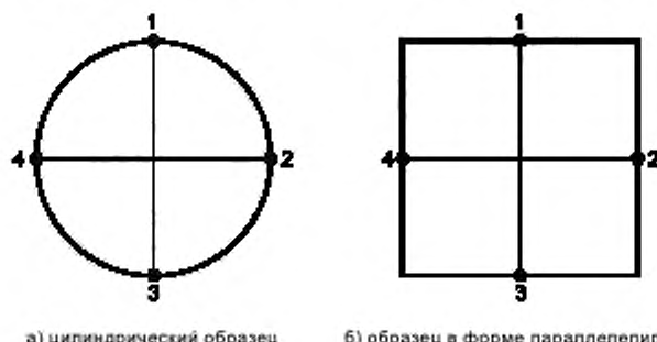
Рисунок 2 — Точки выполнения измерения толщины образца (вид сверху)
