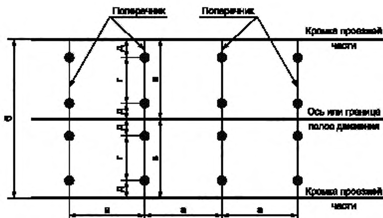
Рисунок 1 — Схема расположения точек измерений толщины слоя геодезическим методом
