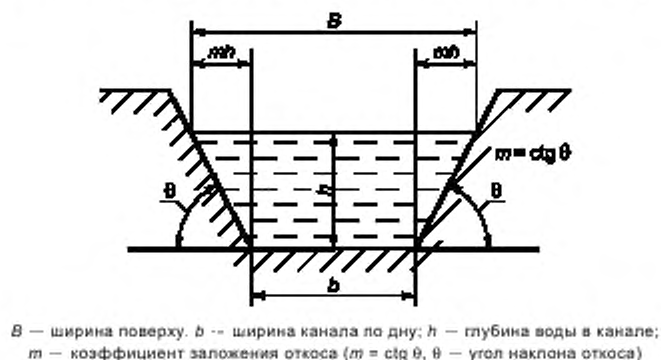
Рисунок 1 — Схема оросительного канала трапецеидального сечения
