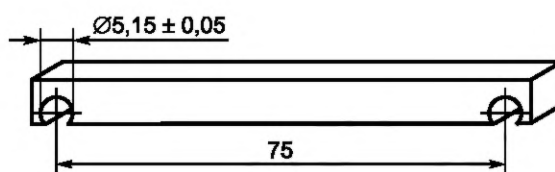
д) Ограничитель движения каретки
