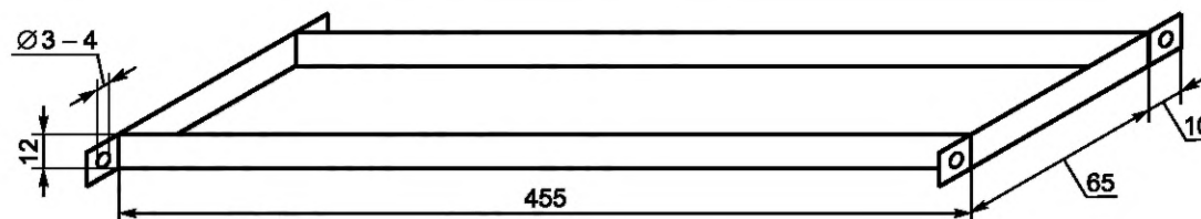
в) Рама для крепления образца
