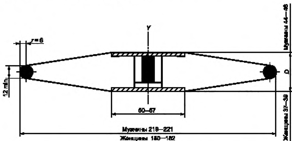
Рисунок 1 — Схема диска
