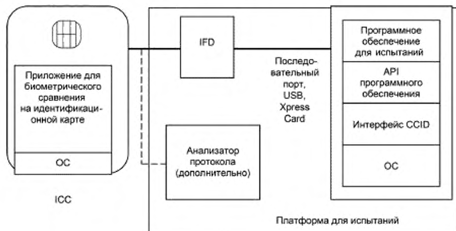
Рисунок В.1 — Обобщенная архитектура испытательной установки
