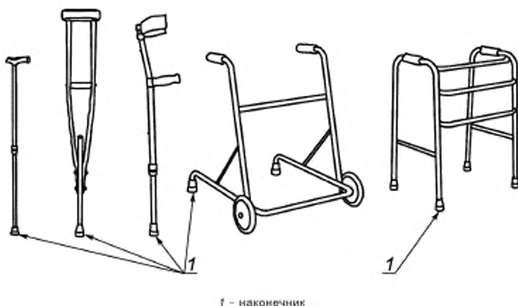
Рисунок 8 — Пример наконечников вспомогательных средств для ходьбы
