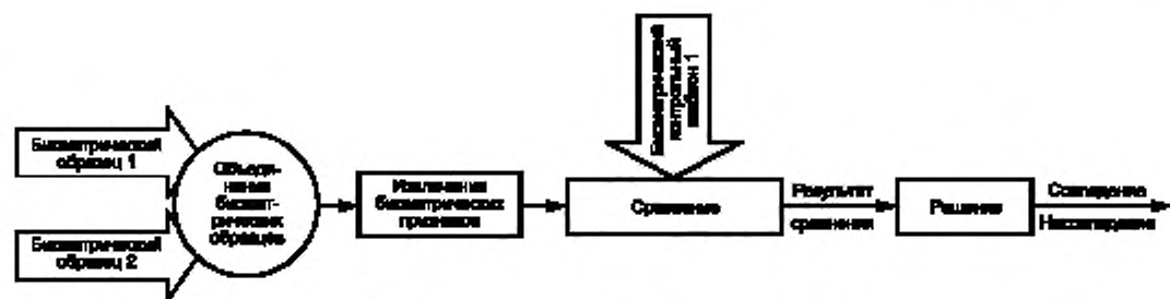
d) Объединение на уровне биометрических образцов
