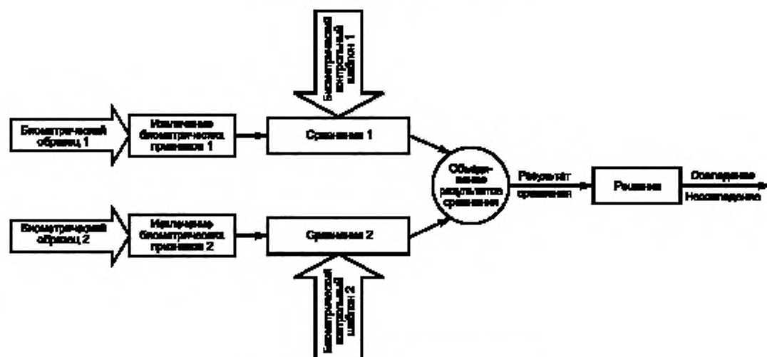
b) Объединение на уровне результатов сравнения
