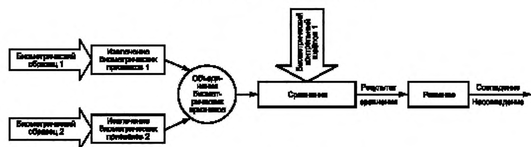
с) Объединение на уровне биометрических признаков
