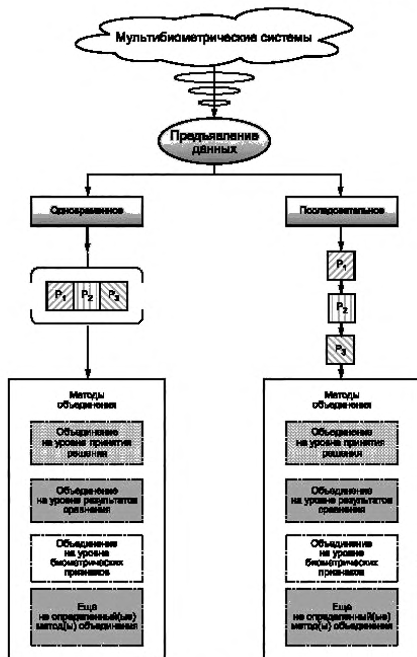
Рисунок 1 — Модель мультибиометрической системы
