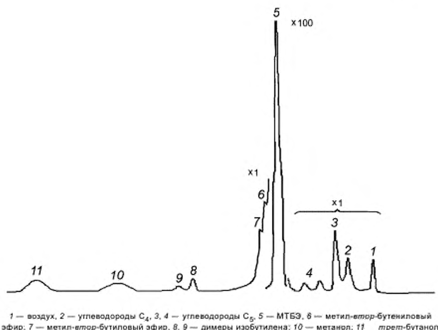
Рисунок 1 — Хроматограмма метил-трет-бутилового эфира на колонке с ТВИН-60
