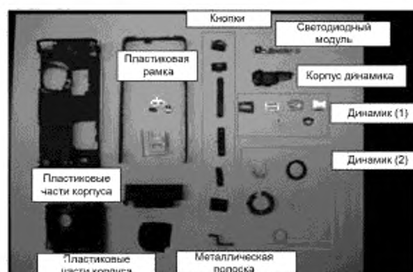
Рисунок Е.5 — Полная разборка нижней части корпуса
