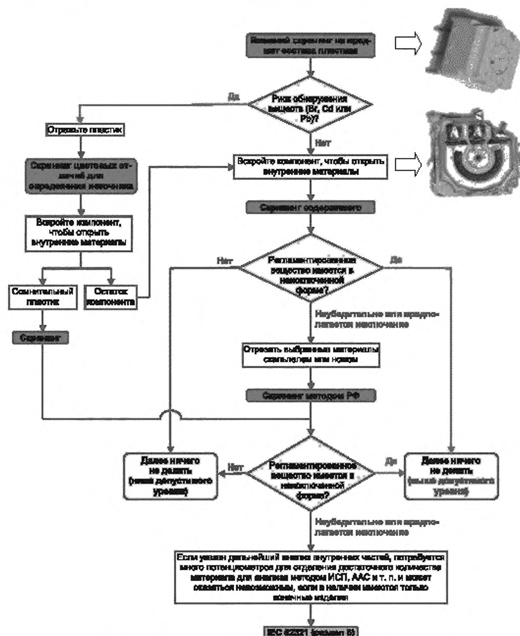
Рисунок A.8 — Отбор образцов компонентов — SMD потенциометр
