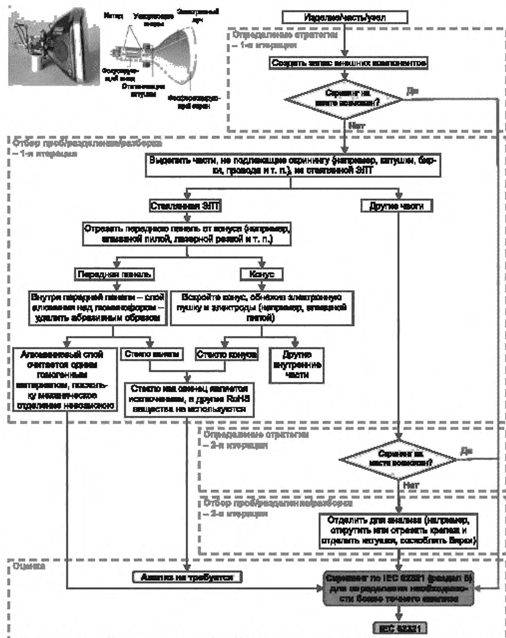
Рисунок А.3 — Отбор образцов ЭПТ
