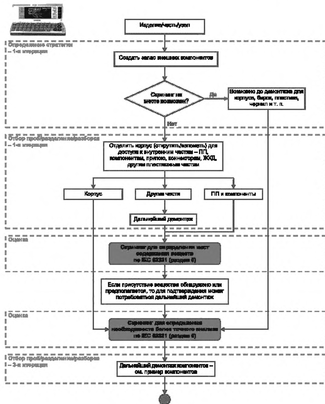
Рисунок A.5 — Отбор образцов PDA/телефона
