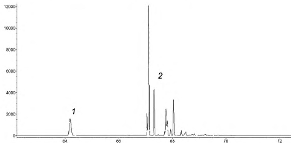
Рисунок В.2 — Типовая хроматограмма автомобильного бензина, содержащего этанол
