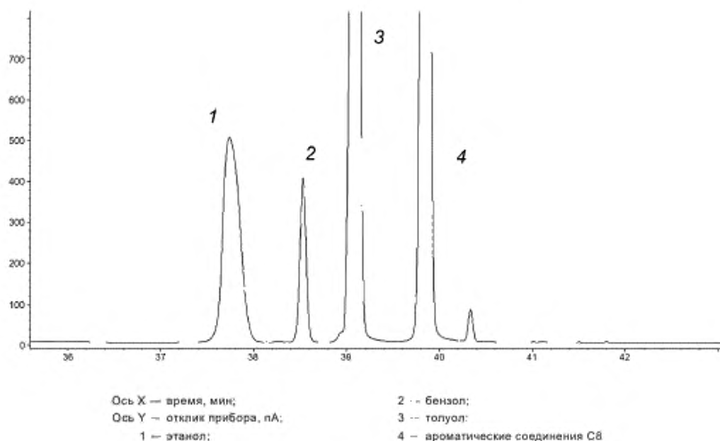
Рисунок В.5 — Расширенная хроматограмма элюирования этанола после его выхода из сульфатной колонки I
