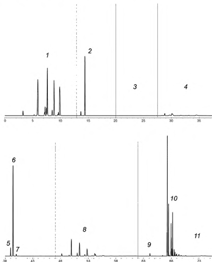
Рисунок В.1 — Типовая хроматограмма автомобильного бензина, содержащего ETBE
