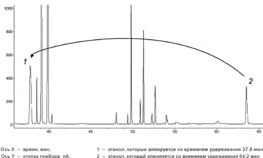
Рисунок В.4 — Хроматограмма, отражающая выход этанола из сульфатной колонки I из-за слишком высокой температуры колонки
