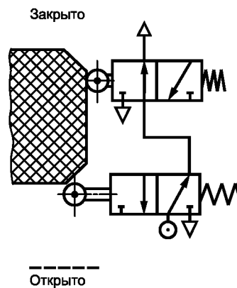
Рисунок L.2 — Два элемента прерывания цепи (клапана)
