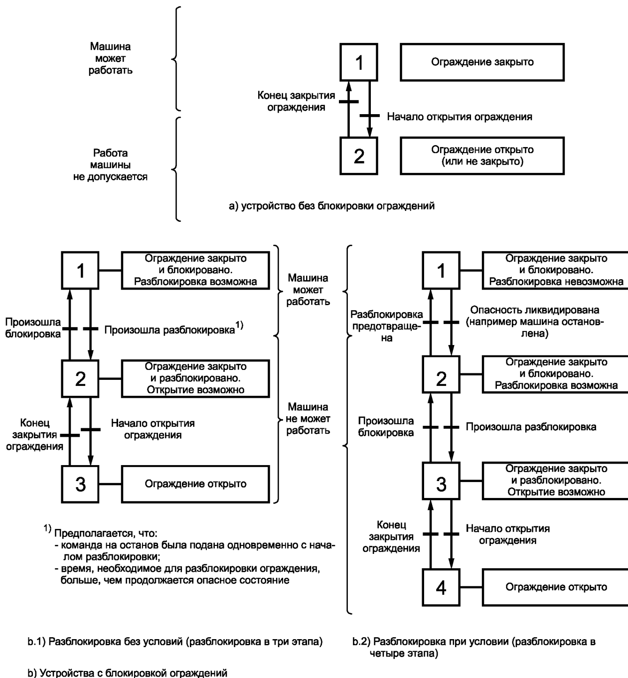
Рисунок 3 — Функциональная схема для различных типов защитных устройств с взаимной блокировкой
