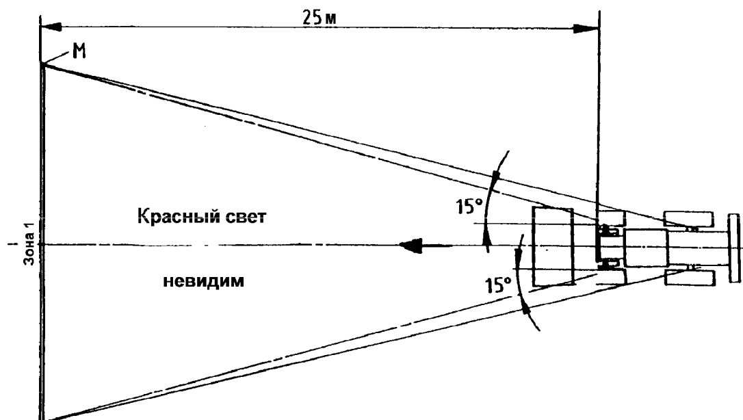
Рисунок В.1 – Видимость огней красного света спереди (4.1.6.1)
