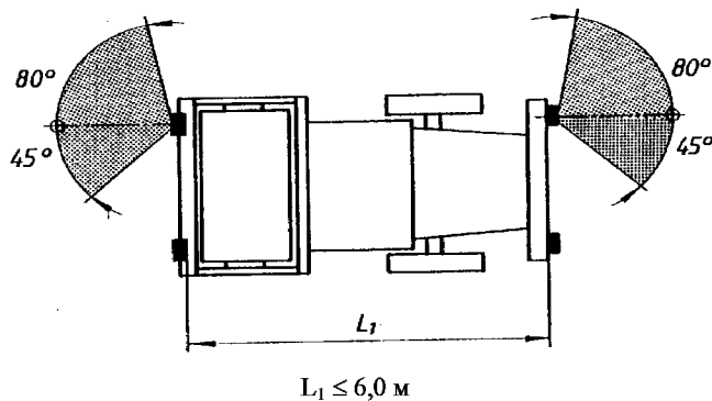
Рисунок Е.5с – Расположение С
