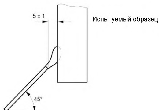
Рисунок 1с – Положение при испытании (пример)
