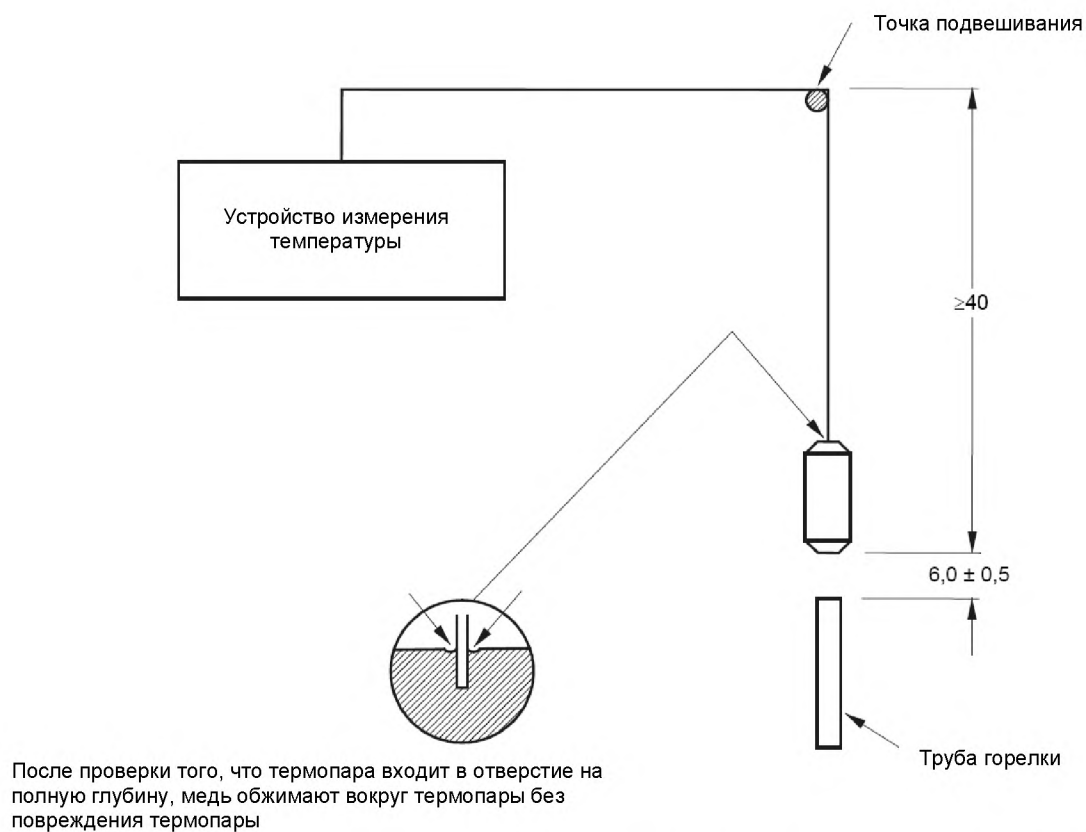
Рисунок А.2 – Установка для подтверждения соответствия
