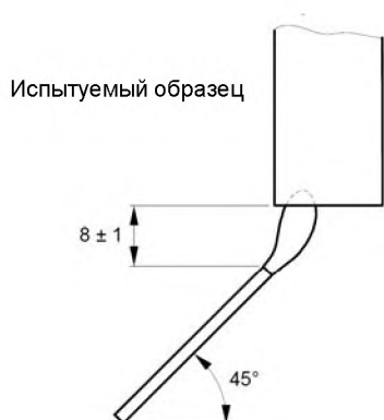
Рисунок 1b – Положение при испытании (пример)
