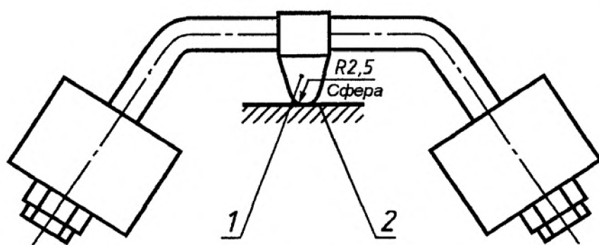
1 – стальной шарик; 2 – испытываемая поверхность
