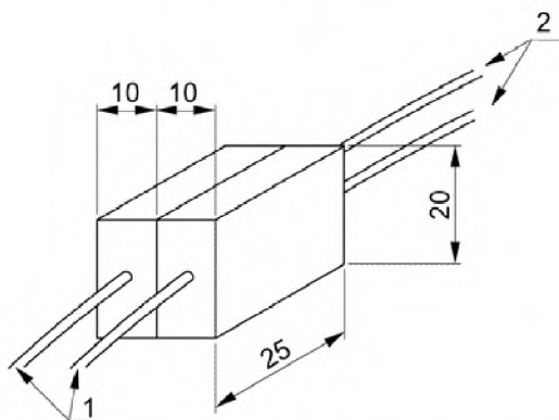
1 – кабель длиной каждой жилы по 10 мм; 2 – монтажные провода светильника
