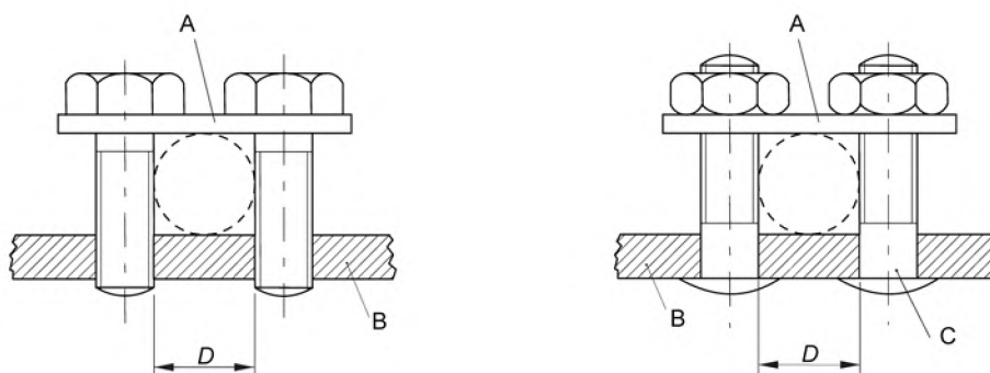
Рисунок 13 – Контактные зажимы с крепежной головкой или крепежной гайкой
