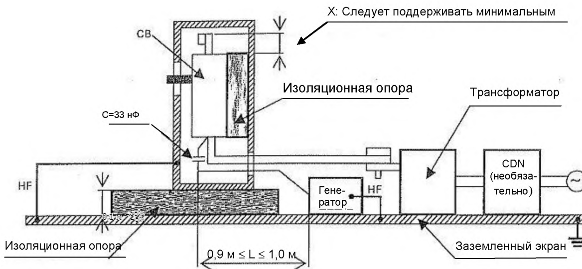
Рисунок F.17 — Схема испытания для проверки устойчивости к электромагнитным полям излучения высокой частоты
