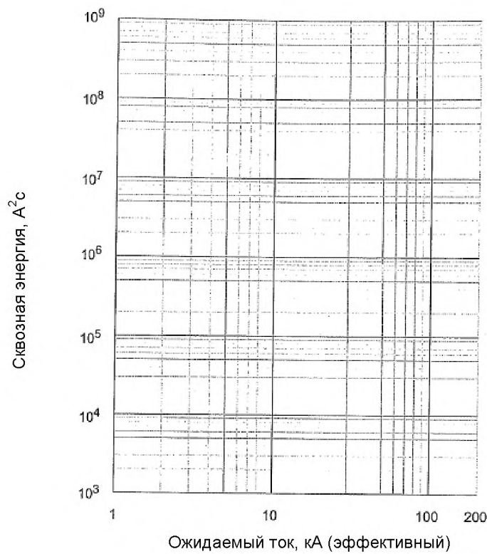
Рисунок К.4 — Шаблон для характеристик сквозной энергии по сравнению с ожидаемым током от 1 до 200 кА
