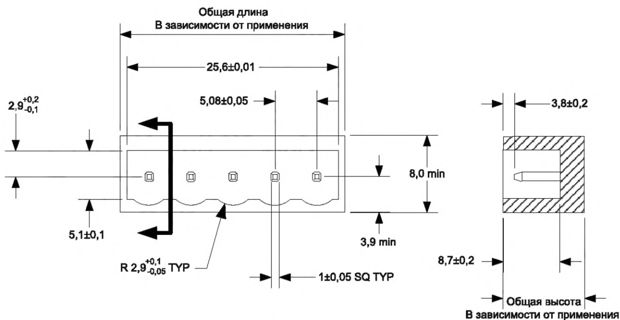
Рисунок 58 — Геометрия открытого разъема
