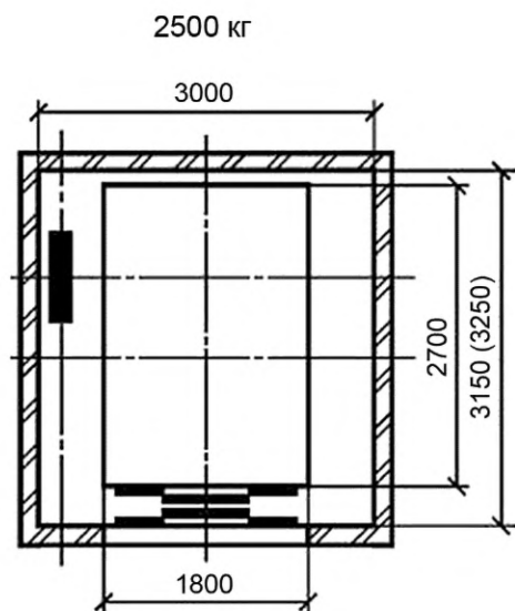
Высота кабины – 2500 Высота дверного проема – 2500
