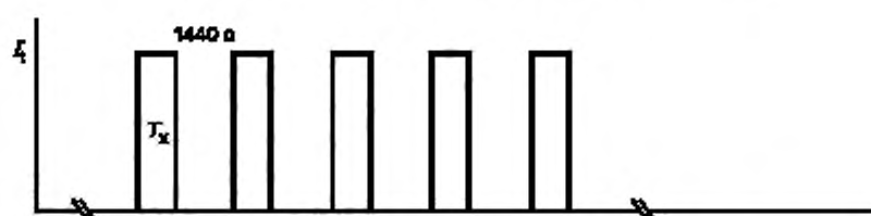
Профиль испытательного тока для AC-52b, AC-53b, AC-58b
