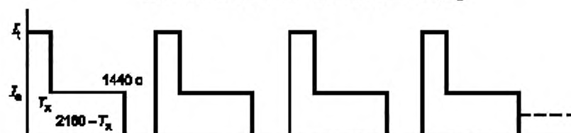
Профиль испытательного тока для AC-52a, AC-53a, AC-58a
