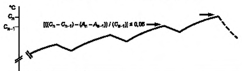
Характерный профиль превышения температуры
