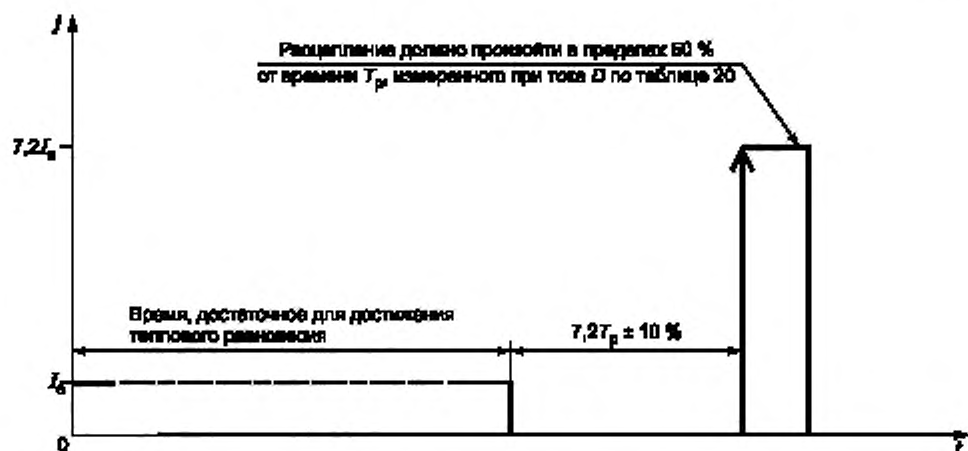
Рисунок 3 — Испытание тепловой памяти
