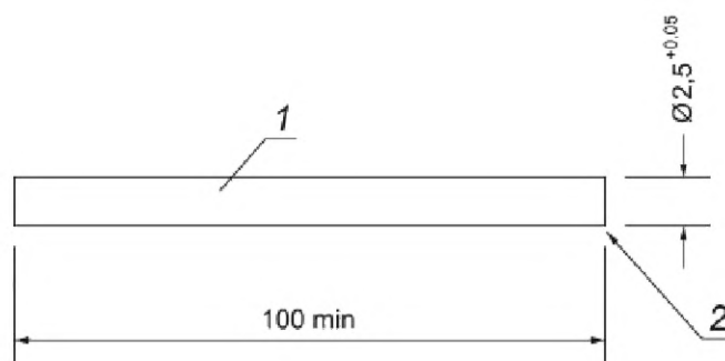
1 — испытательный стержень (металлический); 2 — прямоугольные острые края
