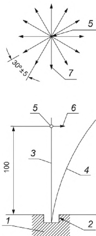
Рисунок 2а) — Принцип устройства установки для испытания на прогиб безвинтовых зажимов
