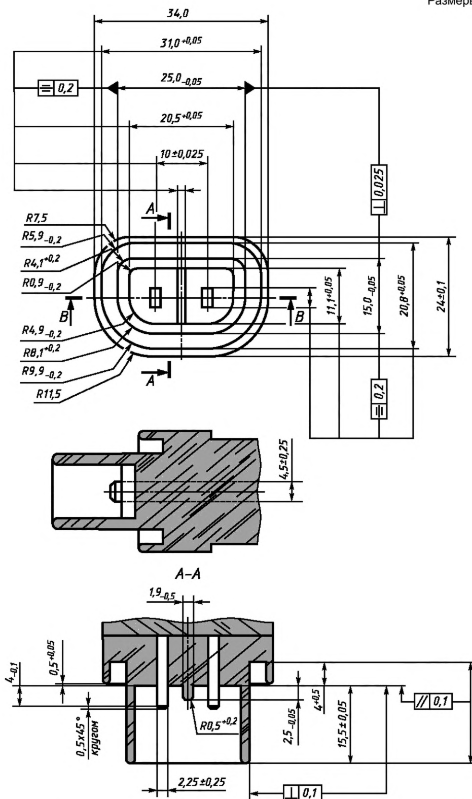
Рисунок 1А — «Проходной» калибр для соединителей согласно стандартному листу С (см. 9.1)
