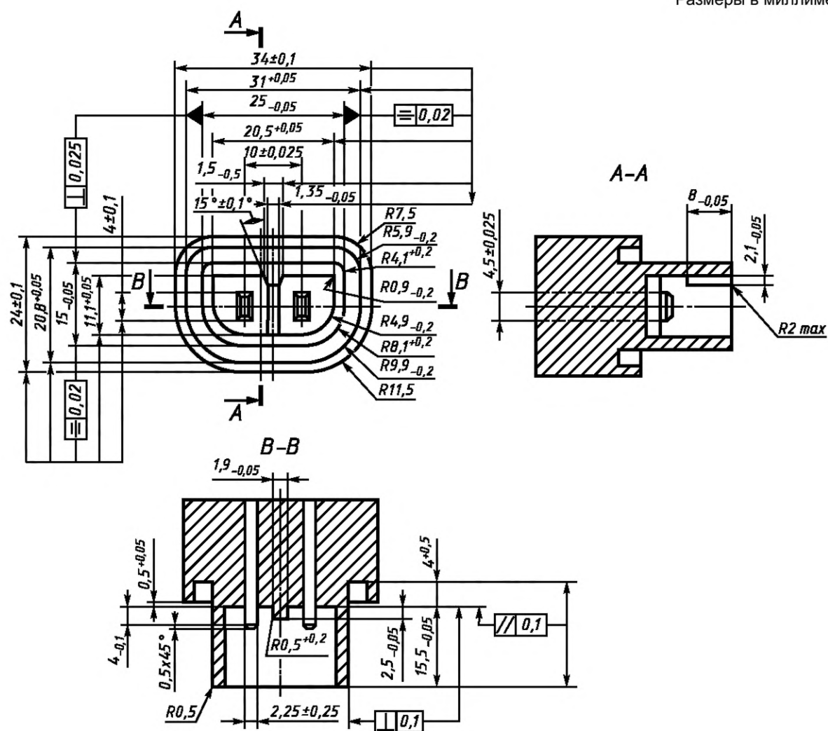
Рисунок 1 — «Проходной» калибр для соединителей согласно стандартному листу А (см. 9.1)
