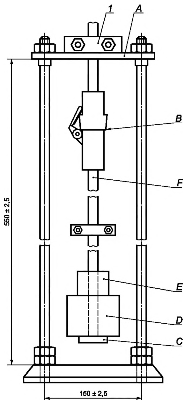
1 — кабельный зажим; A — монтажная плита; B — приборный соединитель; F — кабель; E — дополнительный груз; D — основной груз; C — держатель
