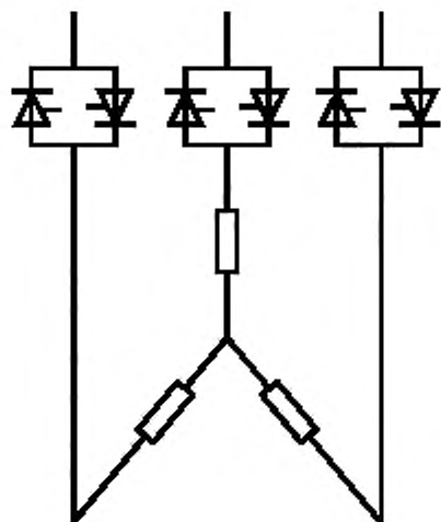
а — Нагрузка со схемой «звезда», тиристоры между нагрузкой и питанием
