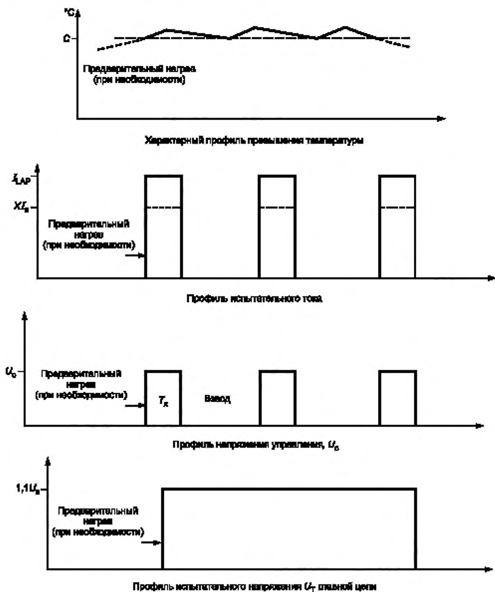
Рисунок F.2 — Профиль испытания на перегрузочную способность
