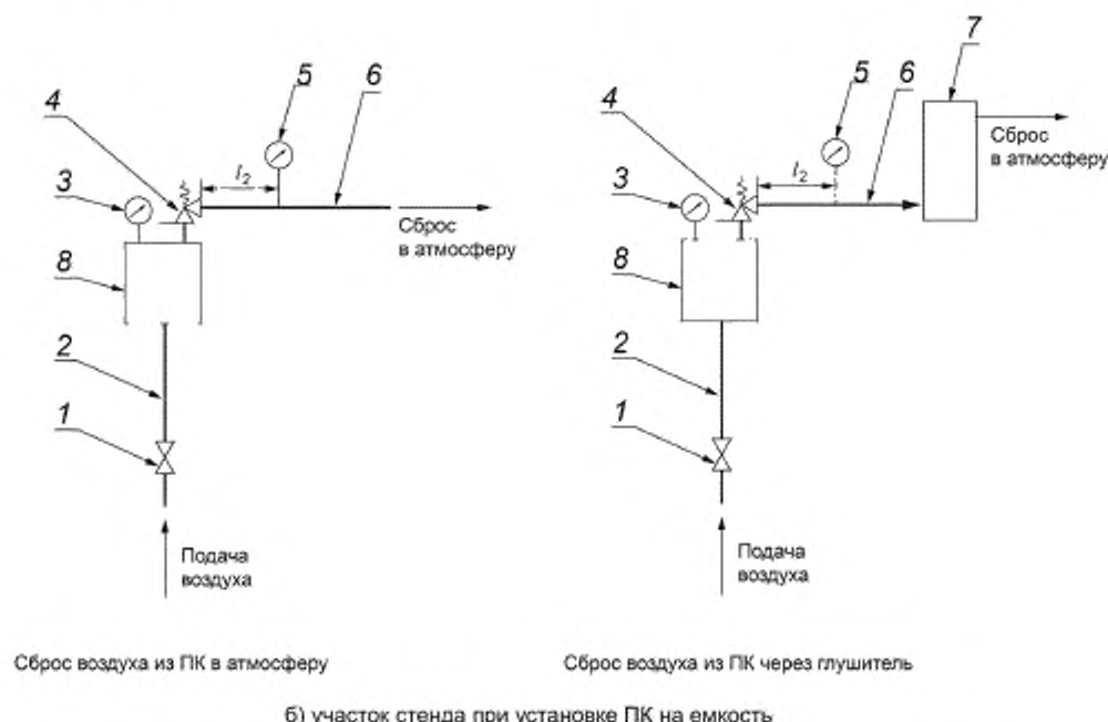
1 — запорный клапан; 2 — трубопровод на входе ПК; 3, 5 — прибор для измерения давления; 4 — испытуемый ПК; 6 — трубопровод на выходе ПК; 7 — глушитель; 8 — емкость
