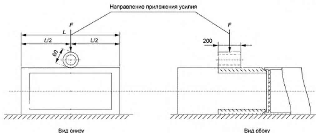
Рисунок 109 — Типовая испытательная установка для механических испытаний основания
