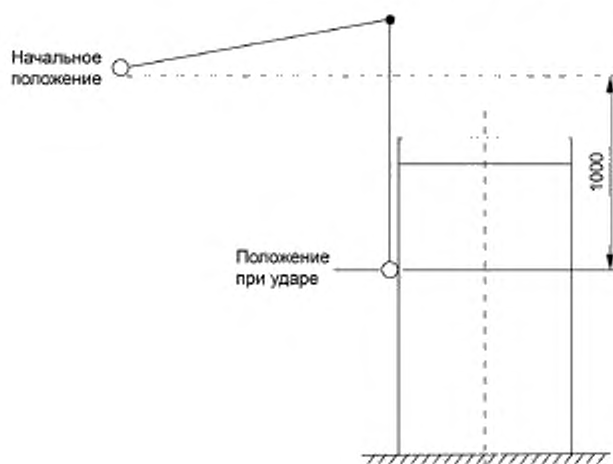
б — Схема проведения испытания для подтверждения стойкости к удару при монтаже НКУ-ОП-Д на земле без фиксации в основании
