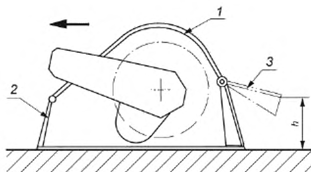
1 — корпус смесительной камеры; 2 — передняя заслонка; 3 — задняя заслонка
