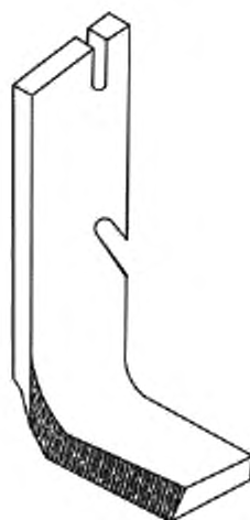
Рисунок А.10 — Рабочий орган типа «L-образный нож»
