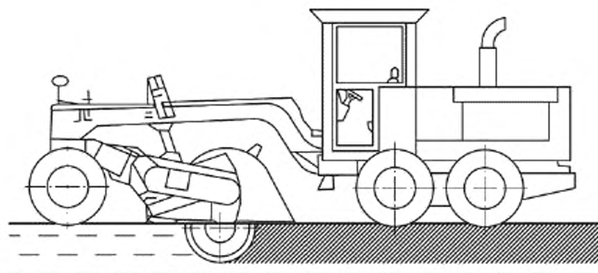
Рисунок А.2 — Стабилизатор грунта на базе автогрейдера с центральным расположением фрезерного барабана с горизонтальной осью вращения
