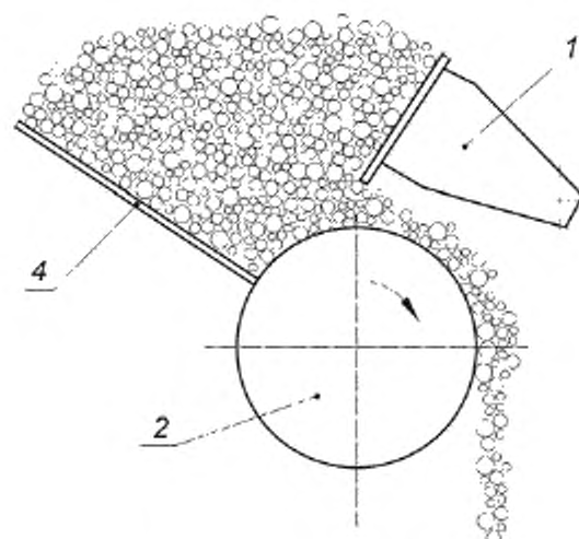
а) с помощью подающего барабана
