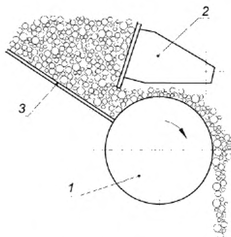
а) с помощью разбрасывающего барабана
