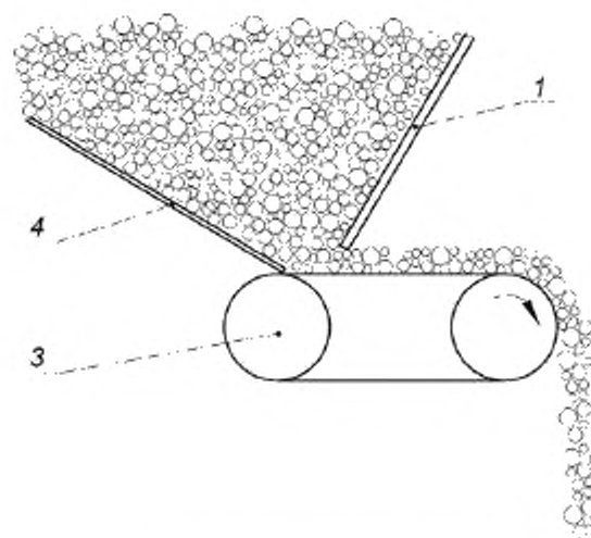
б) с помощью конвейерного питателя
