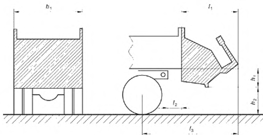
а) в транспортном положении
