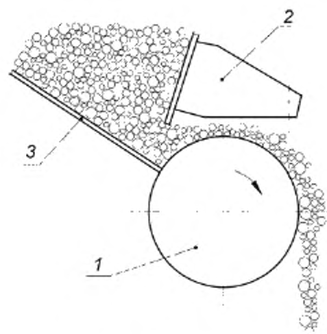
б) под действием сил гравитации
