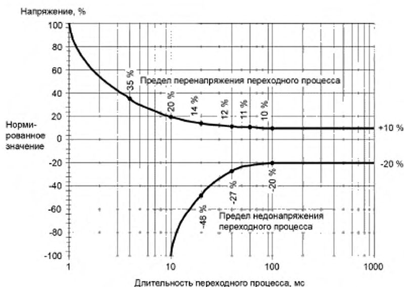
Рисунок В.3 — Допустимые отклонения источника классификации 3
