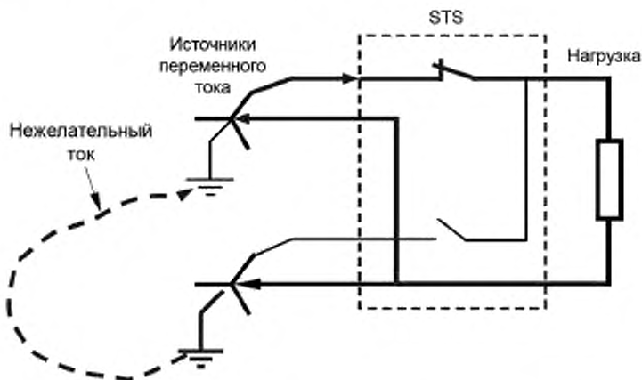
Рисунок 2 — Протекание нежелательного тока нагрузки. Независимое заземление входных источников переменного тока. Общая нейтраль STS
