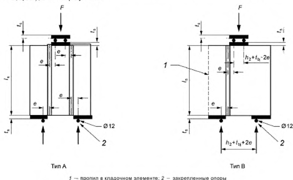
Рисунок Б.2 — Схемы нагружения образцов в зависимости от их типа
