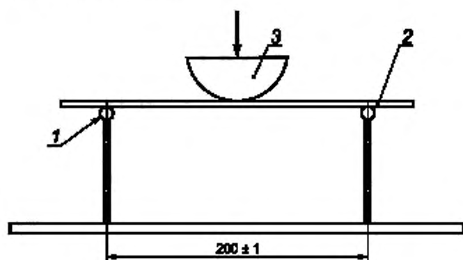
1 — металлические опоры, 2 — образец; 3 — прижим
