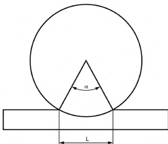
Рисунок A.2 — Определение угла и хорды
