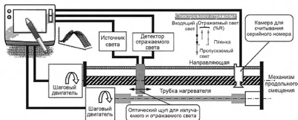
Рисунок A.2.1 — Интерферометр. Общий принцип действия
