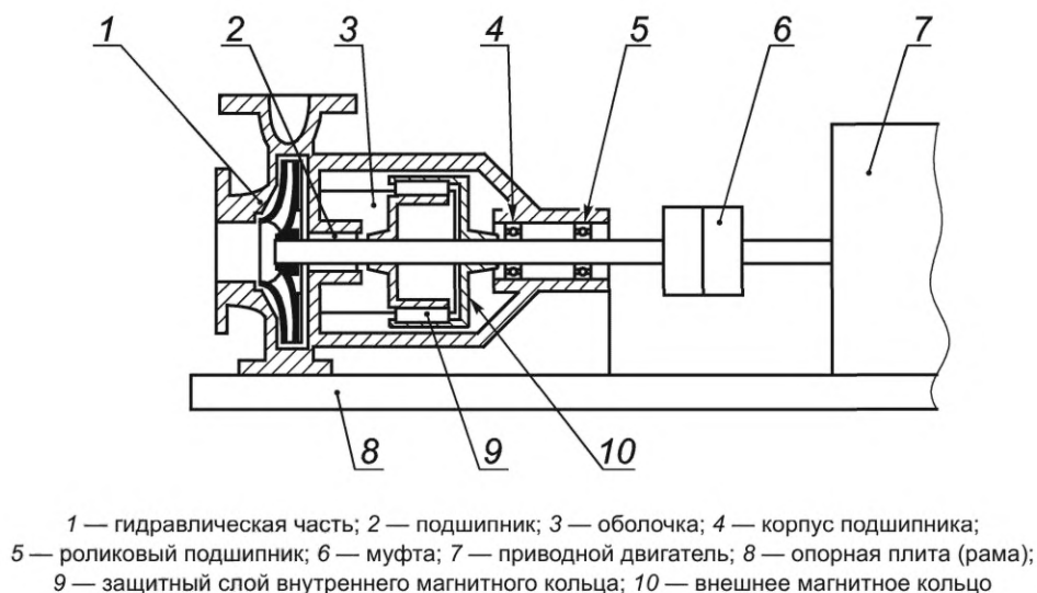
Рисунок 2 — Пример насоса с магнитным приводом (MDP)
