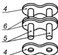
в — наружное звено двухрядное
