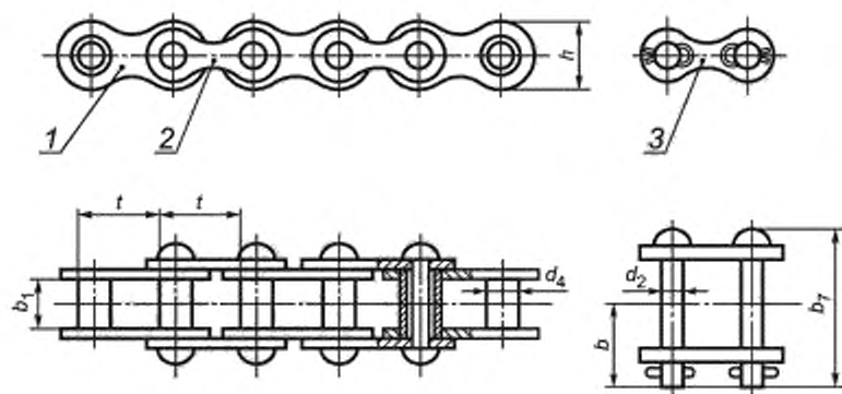
1 — внутреннее звено; 2 — наружное звено; 3 — соединительное звено
