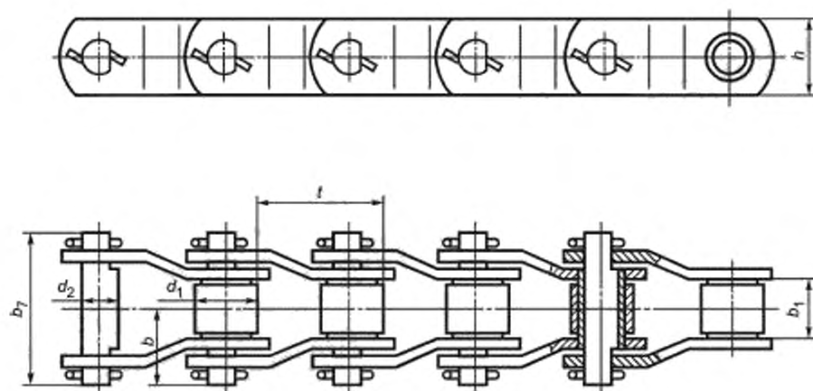
Рисунок 7 — Цепь типа ПРИ
