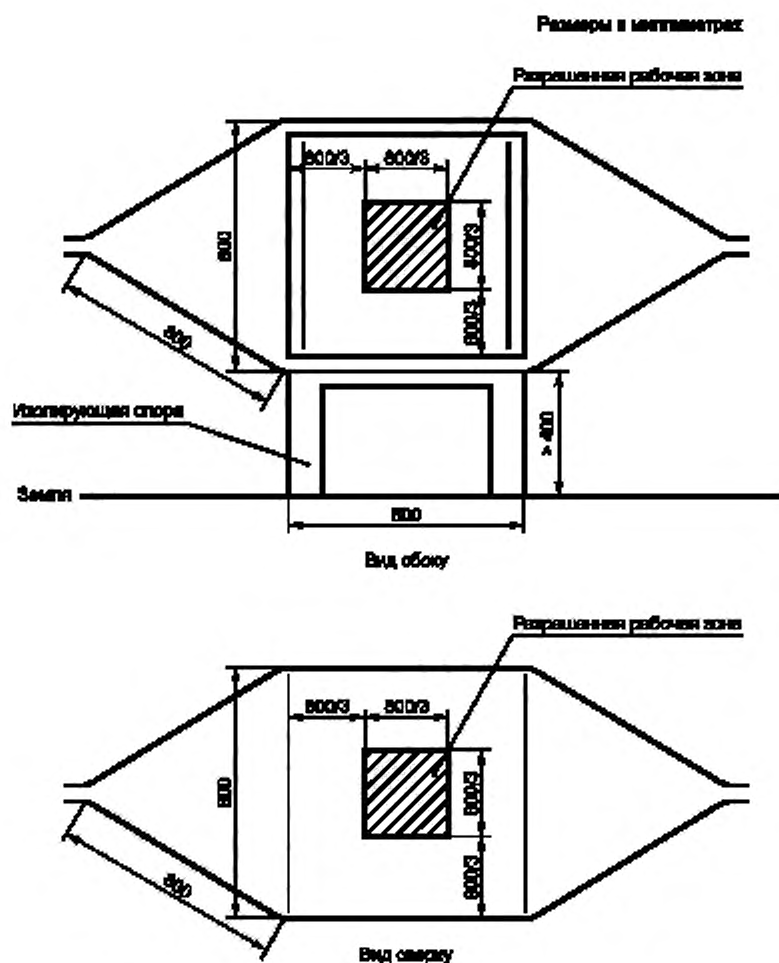
Рисунок 4 – Размеры для 800-миллиметровой полосковой системы
