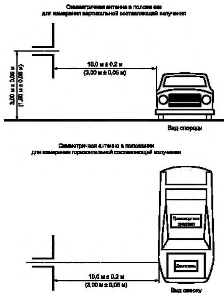
Рисунок 2 — Расположение антенны по отношению к транспортному средству
