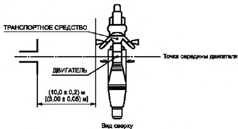
Рисунок 4 — Положение антенны по отношению к транспортному средству
