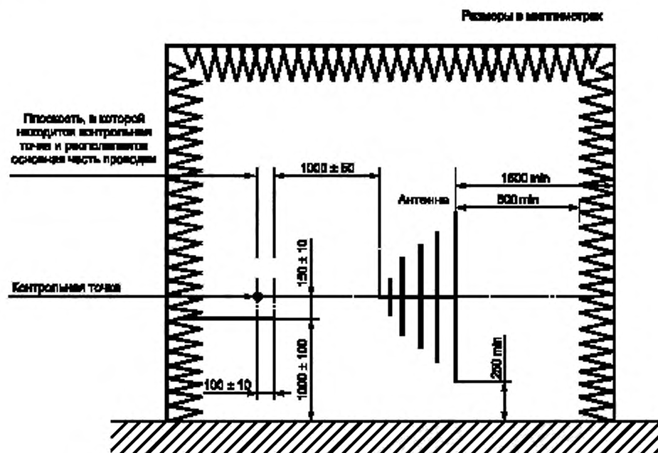
Рисунок 2 — Испытание на устойчивость ЭСУ в условиях свободного поля. Испытательная камера. Вид в плоскости продольной симметрии
