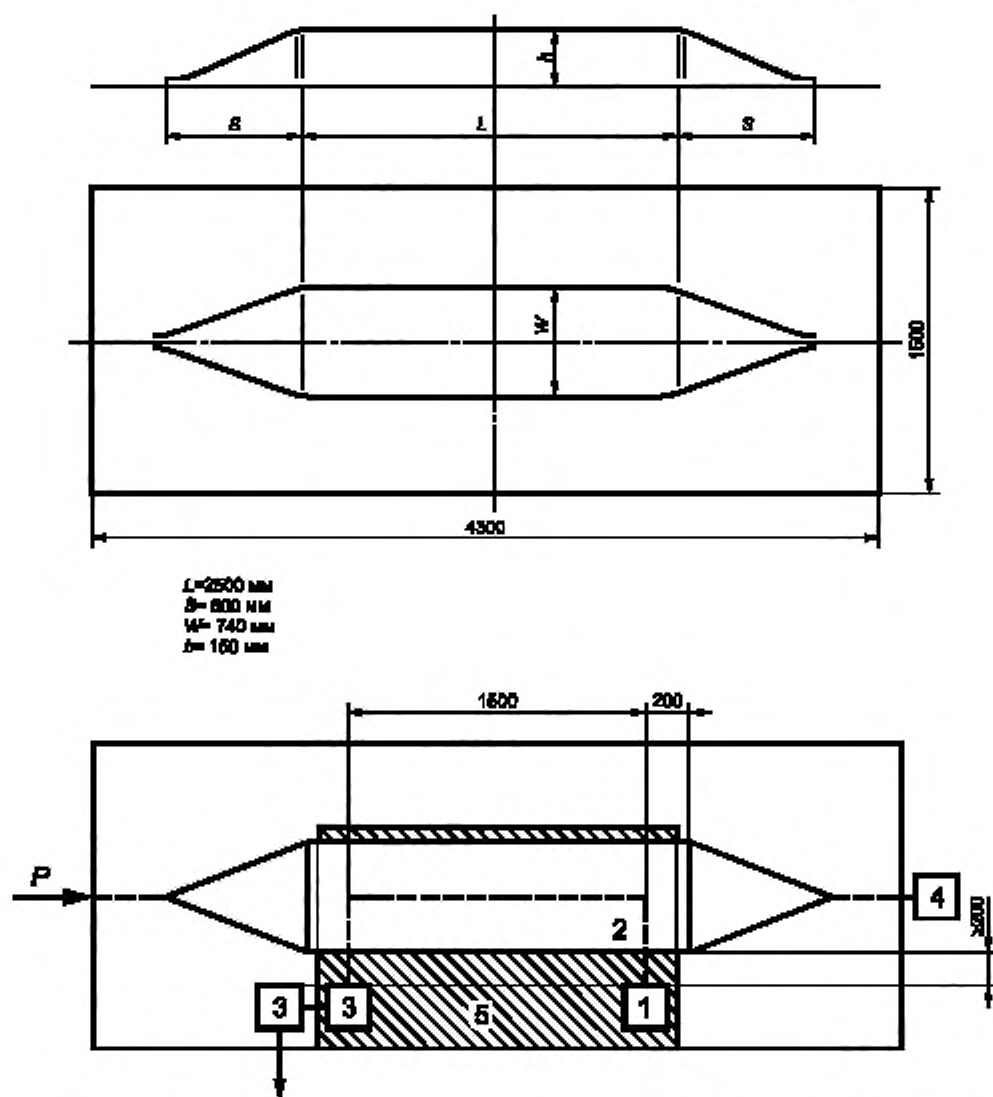
Рисунок 2 – Испытание в 150-миллиметровой полосковой системе
