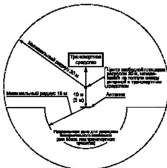
Рисунок 1 — Площадка для испытаний транспортного средства. Горизонтальная площадка, не имеющая поверхностей, отражающих электромагнитные волны
