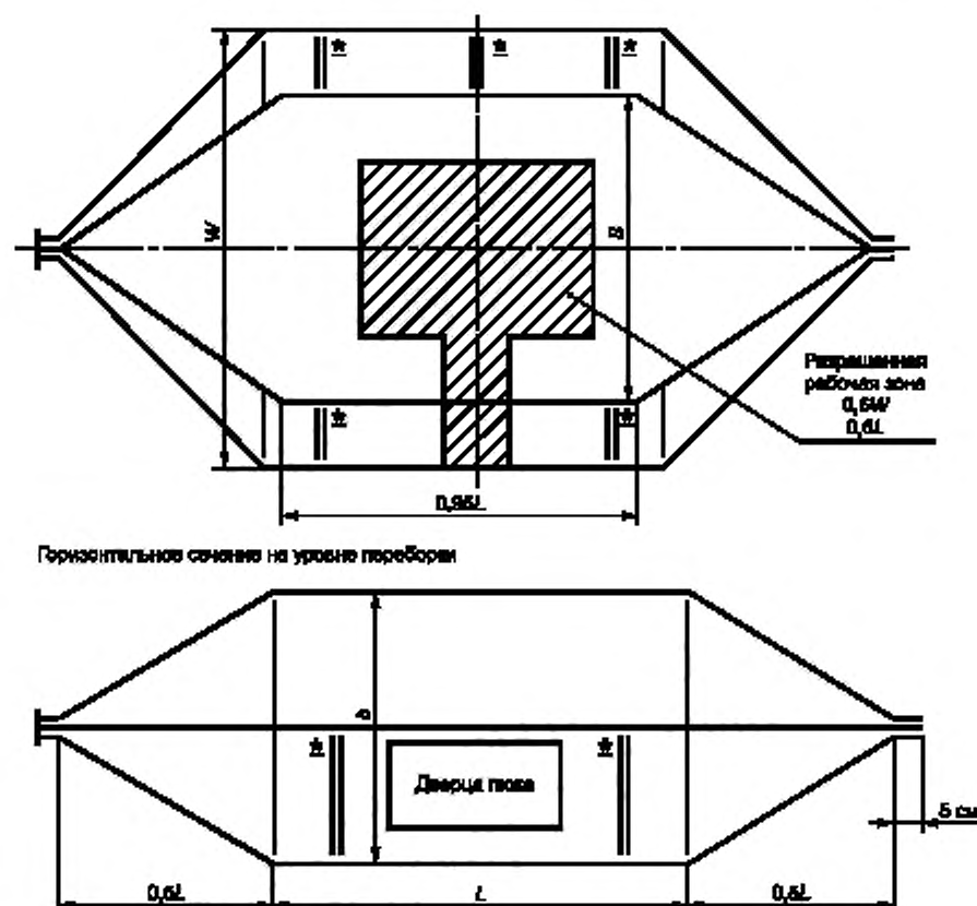
Вертикальное сечение
