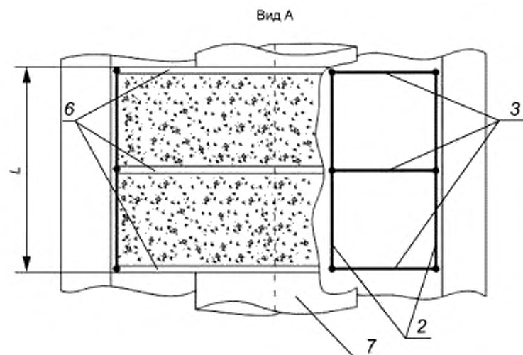
б) вид сверху полимерно-контейнерного балластирующего устройства с увеличенными габаритными размерами и массой, заполненного насыпным грунтом и установленного на трубопровод
