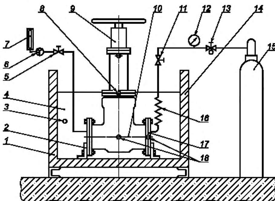
1 — опорные кронштейны; 2 — изоляция; 3 — термopара охлаждающей среды; 4 — охлаждающая среда; 5, 11 — запорная арматура; 6 — термopара (температура телия на выходе); 7 — расходомер; 8 — термopара на корпусе/фланце крышки; 9 — испытуемая арматура; 10 — термopара внутри арматуры; 12 — манометр; 13 — регулятор давления; 14 — охлаждающий бак; 15 — баллон с испытательной средой; 16 — змеевик; 17 — глухой фланец; 18 — термopара на корпусе (по требованию заказчика) и на глухом фланце.
