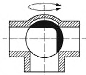
Рисунок А.4 — Вертикальный тип, L-образное отверстие
