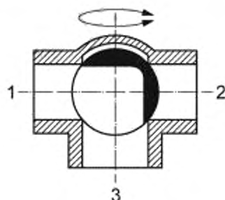
Рисунок А.7 — Ходы 1 и 3 соединены, ход 2 закрыт
