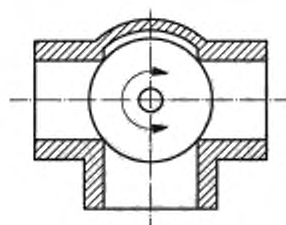
Рисунок А.1 — Горизонтальный тип
