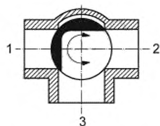
Рисунок А.11 — Ход 1 закрыт, ходы 2 и 3 соединены
