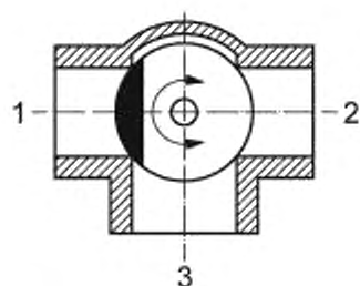
Рисунок А.15 — Ход 1 закрыт, ходы 2 и 3 соединены
