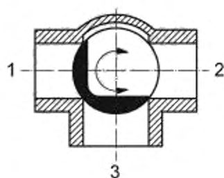
Рисунок А.12 — Кран закрыт
