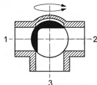
Рисунок А.8 — Ходы 2 и 3 соединены, ход 1 закрыт
