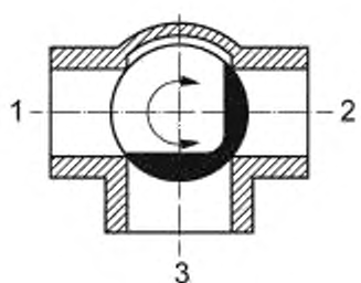
Рисунок А.13 — Кран закрыт
