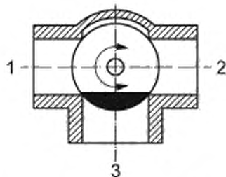
Рисунок А.16 — Ход 3 закрыт, ходы 1 и 2 соединены
