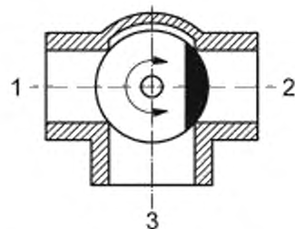
Рисунок А.17 — Ход 2 закрыт, ходы 1 и 3 соединены
