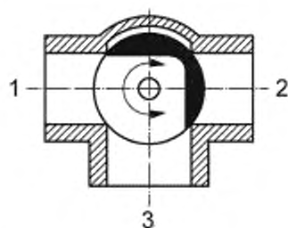
Рисунок А.10 — Ход 2 закрыт, ходы 1 и 3 соединены
