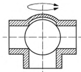
Рисунок А.2 — Вертикальный тип
