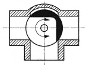
Рисунок А.3 — Горизонтальный тип, L-образное отверстие
