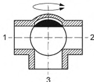
Рисунок А.9 — Ходы 1, 2 и 3 соединены
