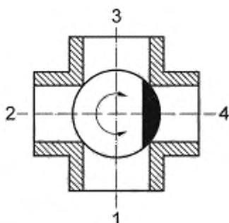
Рисунок А.18 — Ходы 1, 2 и 3 соединены, ход 4 закрыт
