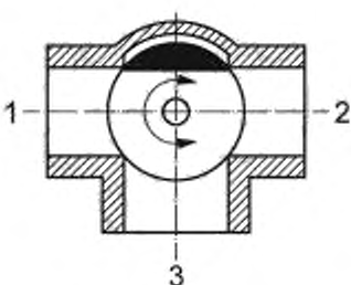
Рисунок А.14 — Ходы 1, 2 и 3 соединены
