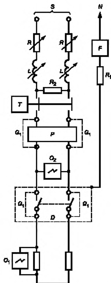
S — источник питания; R — регулируемый резистор нагрузки; L — регулируемая катушка индуктивности нагрузки; T — замыкающее устройство; F — медный проволочный предохранитель; R_1 — резистор ограничения тока повреждения; R_2 — резистор, отводящий ток 10 А на фазу; P — УЗКЗ; G_1 — временное калибровочное соединение; O_1 — датчик тока; O_2 — датчик напряжения; D — испытуемый разъединитель
