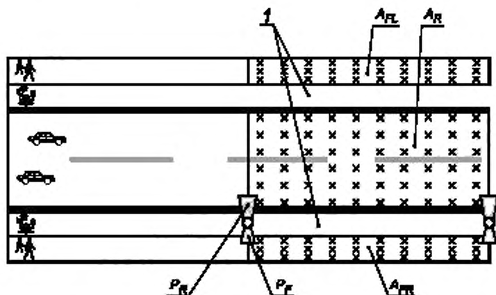
A_R , A_{FL} и A_{FR} — элементы расчетного поля: проезжая часть, левая и правая пешеходные дорожки соответственно; P_R и P_F — ОП, направленные на проезжую часть и правую пешеходную дорожку соответственно; 1 — полосы газона; значками «x» показаны расчетные точки на расчетном поле
