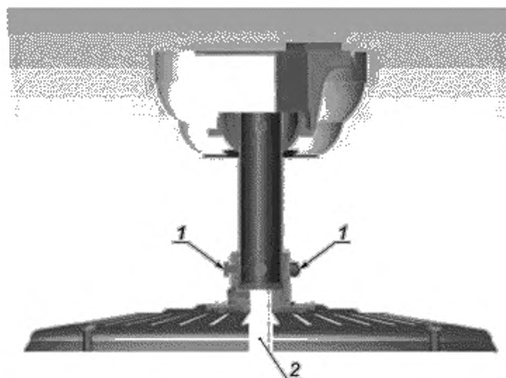
1 — стопорные винты; 2 — направленный вниз шток с резьбой
