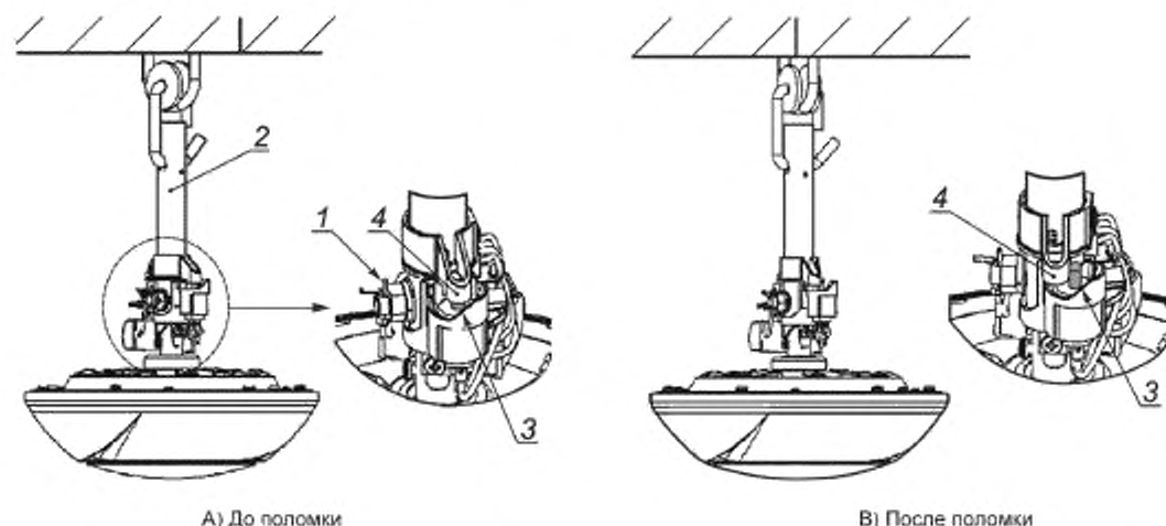
А — Система подвеса (определение 3.102): 1 — соединительный болт; 2 — монтажный шток; В — Устройство, отключающее вентилятор от сети питания перед поломкой системы подвеса: 3 — электрическое устройство защиты (защитный выключатель), закрепленное на блоке двигателя для отключения подачи питания перед поломкой соединительного болта; 4 — стопор, закрепленный на монтажном штоке, для поддержания защитного выключателя в исходном положении «включено»
