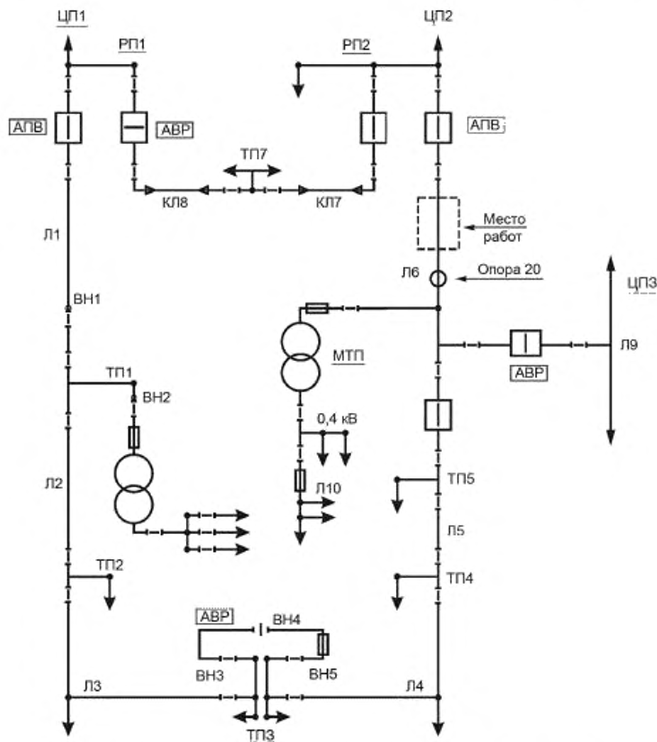
Рисунок Ж.2 — Схема участка распределительной электросети 6—10 кВ, секционированной в трансформаторной подстанции ТПЗ в нормальном режиме работы
