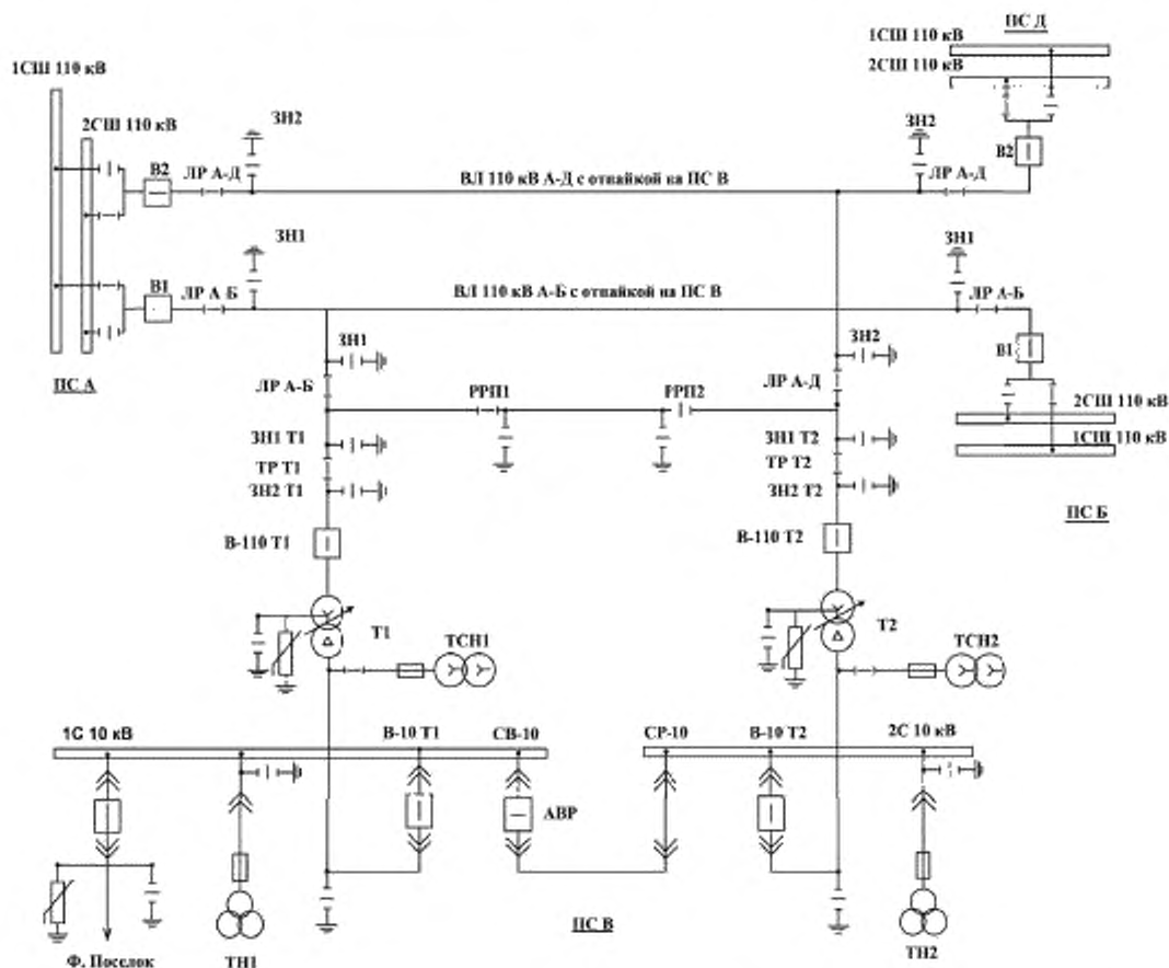
Рисунок Г.1 — Участок сети напряжением 110 кВ с отпавной двухтрансформаторной подстанцией, питающейся от двух транзитных линий электропередачи
