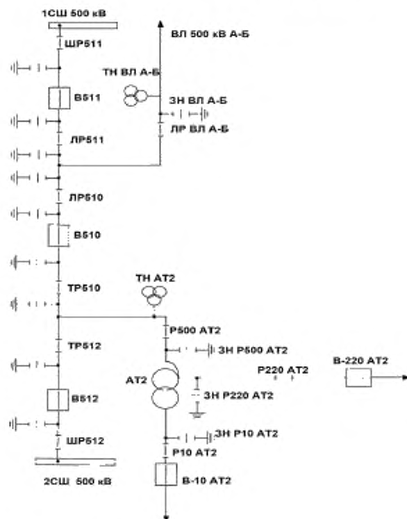
Рисунок Е.3 — Схема подстанции 500 кВ, выполненной по полумоторной схеме
