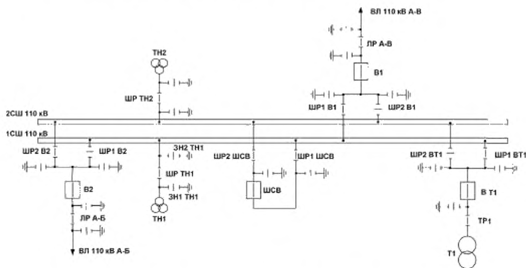
Рисунок Е.1 — Схема распределительного устройства с двумя системами шин
